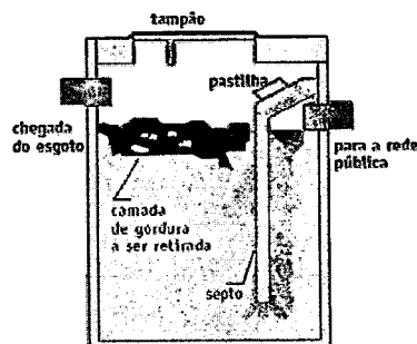
Caixa de Gordura esquema de funcionamento
